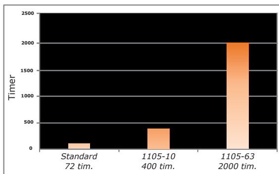
Ozontest: iht. EN 27326, 40°C, 50 pphm
