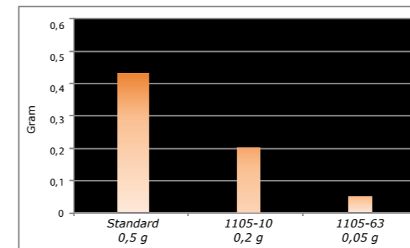
Slitasjetest: iht. ISO 6945, 2000 sykluser, 25N
